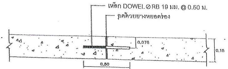
EXPANSION JOINT ทุกระยะไม่เกิน 100 ม. NOT TO SCALE
