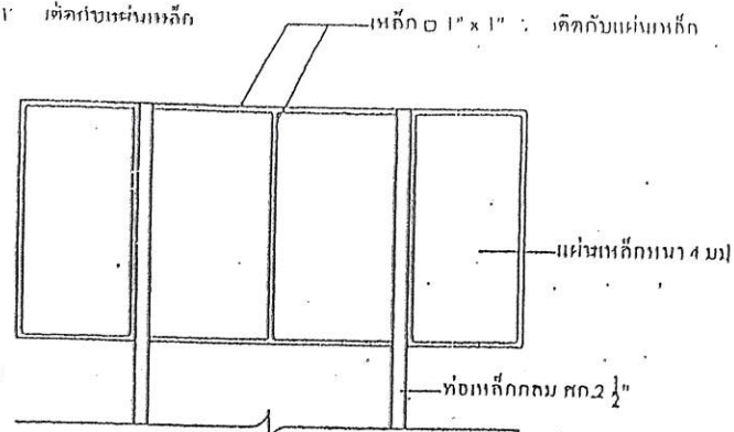
รูปด้านหลัง มาตราส่วน 1:20
