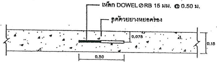
CONTRACTION JOINT ทุกระยะไม่เกิน 10 ม. NOT TO SCALE
