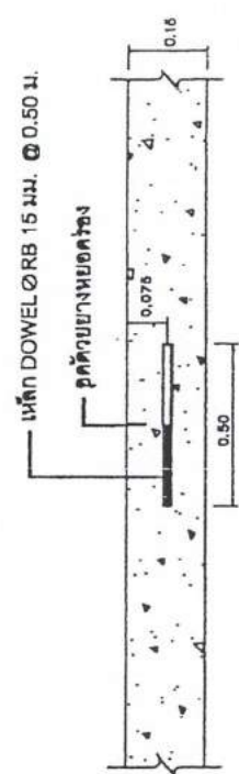
CONTRACTION JOINT NOT TO SCALE ทุกระยะไม่เกิน 10 ม.
